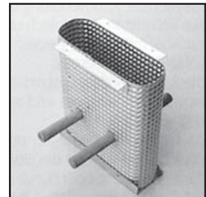
Schalbox mit 2 Ankerstäben
